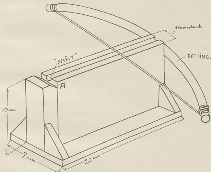
Bild 6. "Belägringskanon" för nedskjutning av fästningsmurar.
