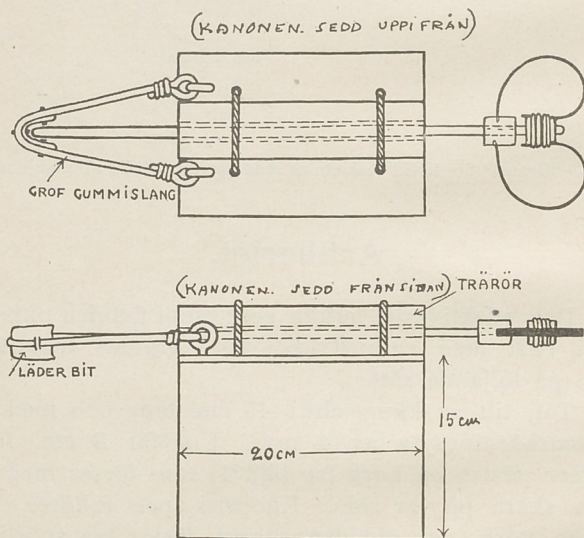
Bild 2. Kanon för direkt beskjutning med "granaten" inlagd, färdig till avskjutning.
