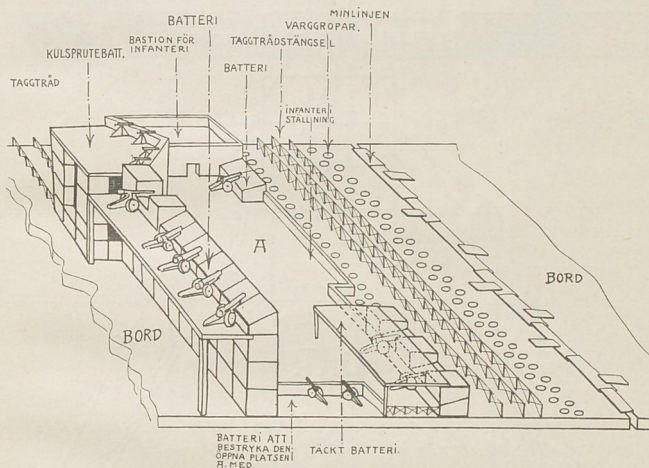
Bild 12. Plan över en fästning.
