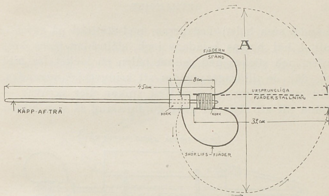
Bild 1. "Granat" för direkt beskjutning sedd uppifrån färdig till avskjutning.
